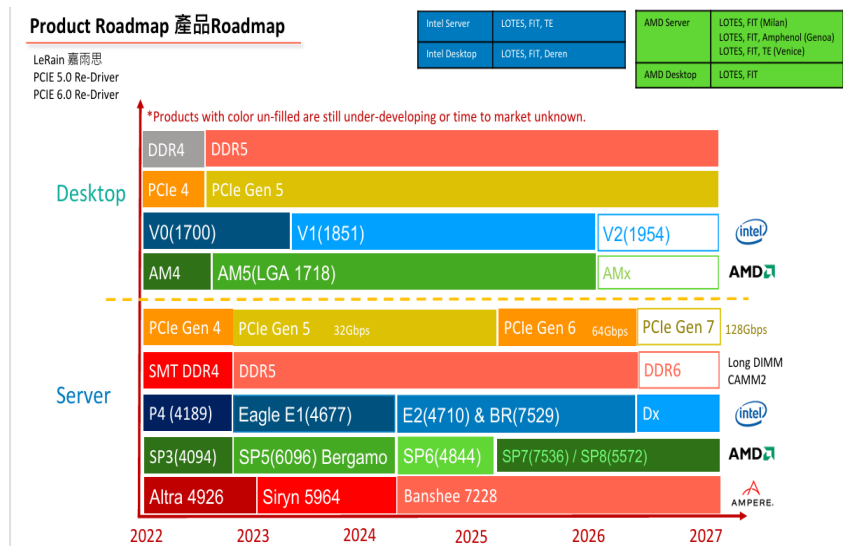
圖九、產品演進，CPU Socket 針腳數持續增加
